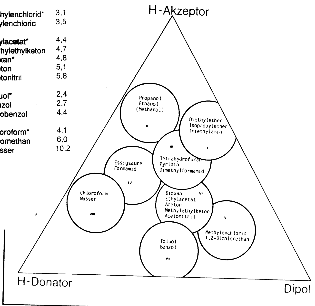
Abb.5: Selektivitätsdreieck
